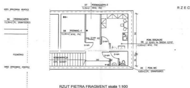
Rzut zaplecza
