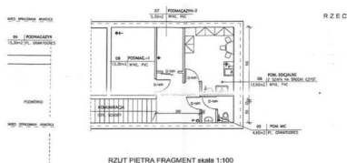
Rzut zaplecza
